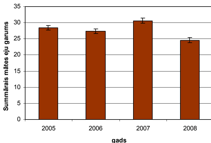
3.2.1.2.attēls. Vidējais summārais mātes eju garums laikā no 2005.g. līdz 2008.gadam svaigi gāztās un lauztās eglēs.
