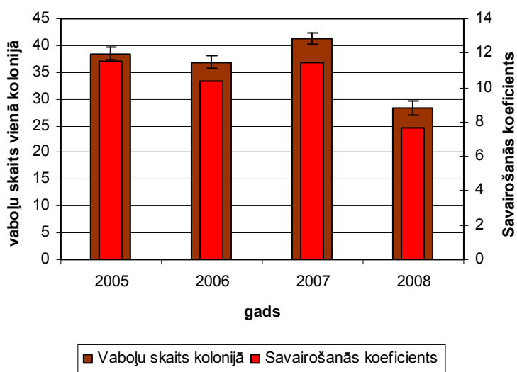
3.2.1.1.attēls. Vidējais jauno vaboļu iznākums un savairošanās koeficients laikā no 2005.g. līdz 2008.gadam svaigi gāztās un lauztās eglēs.
